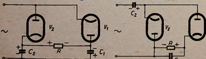
Abb. 3. Greinacher Schaltung Zeichnungen: Hennig
