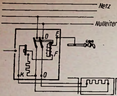
Abb. 3b. Anschluß an Wechselstrom
