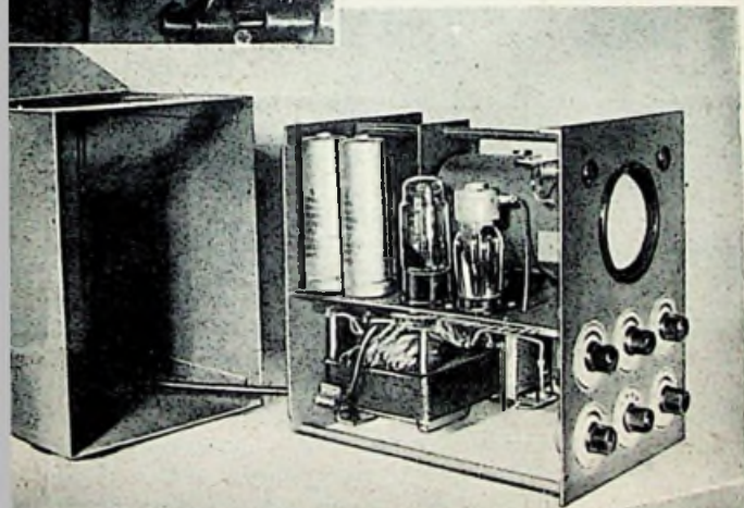
Unten: Ein als Meisterstück eingereichter Katodenstrahlzillograph
