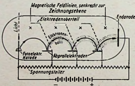
Abb. 2. Grundsätzlicher Aufbau einer Elektronenvervielfacherröhre zum Verstärken des von einer lichtelektrischen Katode gelieferten Elektronenstromes Zeichnungen: Trester
