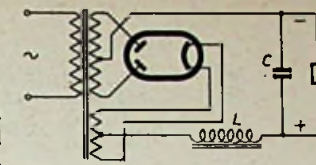
Abb. 5. Drosselspule nach dem Gleichrichter
