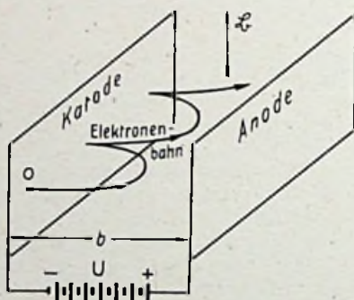
Abb. 1. Zykloidenbahn eines Elektrons in rechtwinklig gekreuzten Feldern. Ausgangspunkt bei 0 aus Ruhelage
